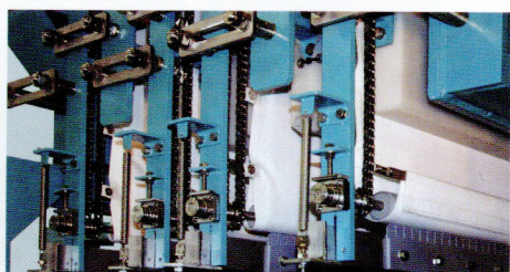
3 移動用ろ布はエンドレス構造のチェーンに取り付けられ、回転とスクレーパーによりケーキを剥離します。
