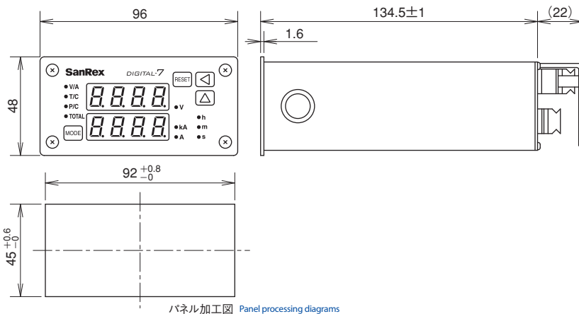
パネル加工図 Panel processing diagrams
